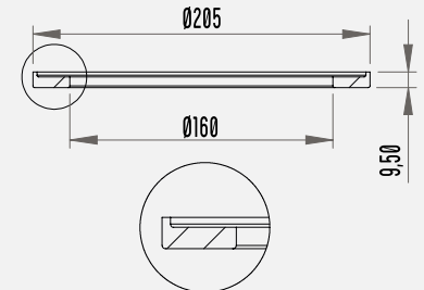
ÖC.045 30 Lt. Düz Güğüm Kapağı Contası - 30 Lt. Flat Bucket Lid Gasket
