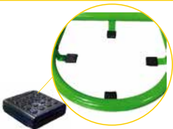
ÖC.287 Güğüm Saşe Pabucu Bucket-Chassis Shock Absorber
