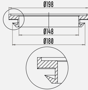
ÖC.042-1 30 Lt. Güğüm Kapağı Contası PVC - 30 Lt. Bucket Lid Gasket PVC
