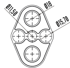
ÖC.137-1 Küçükbaş Sağım Başlığı Hortum Tutucu - Sheep Milking Cluster Hose Holder
