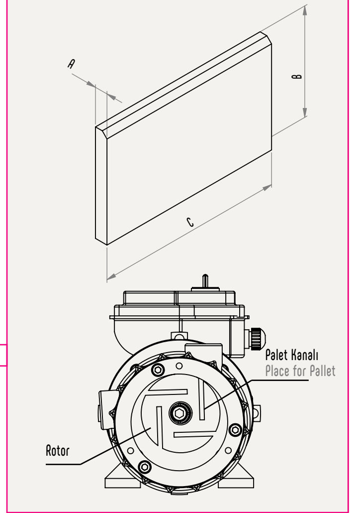
Palet Kömür Takımı 4 Adettir. Pallet Graphite Set (4 Pcs.)
