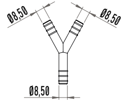
ÖC.137-1 Küçükbaş Sağım Başlığı Hortum Tutucu - Sheep Milking Cluster Hose Holder
