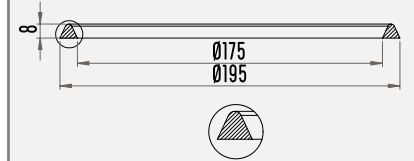
ÖC.044-1 30 Lt. Düz Güğüm Kapağı Beyaz Contası - 30 Lt. Flat Bucket Lid White Gasket
