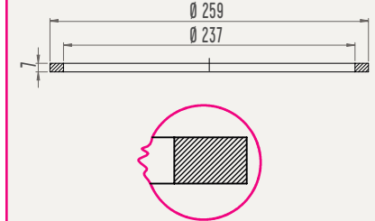
ÖC.050 Vakum Tank Kapağı Contası (Kauçuk) - Vacuum Tank Lid Gasket (Rubber)
